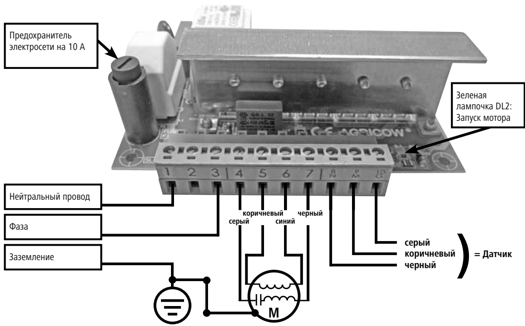
Рисунок 5.2: Схема электрических подключений для моделей CowCleaner Swing до 2015 г.
