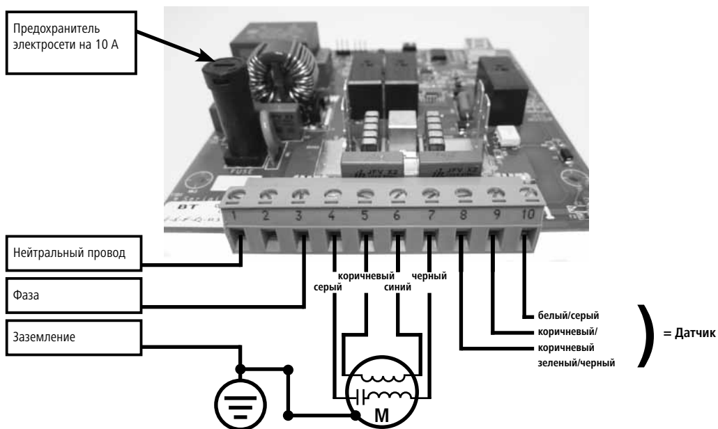
Рисунок 5.2: Схема электрических подключений для моделей CowCleaner Swing до 2015 г.
