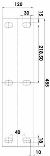
Afbeelding 2: Boorsjabloon
