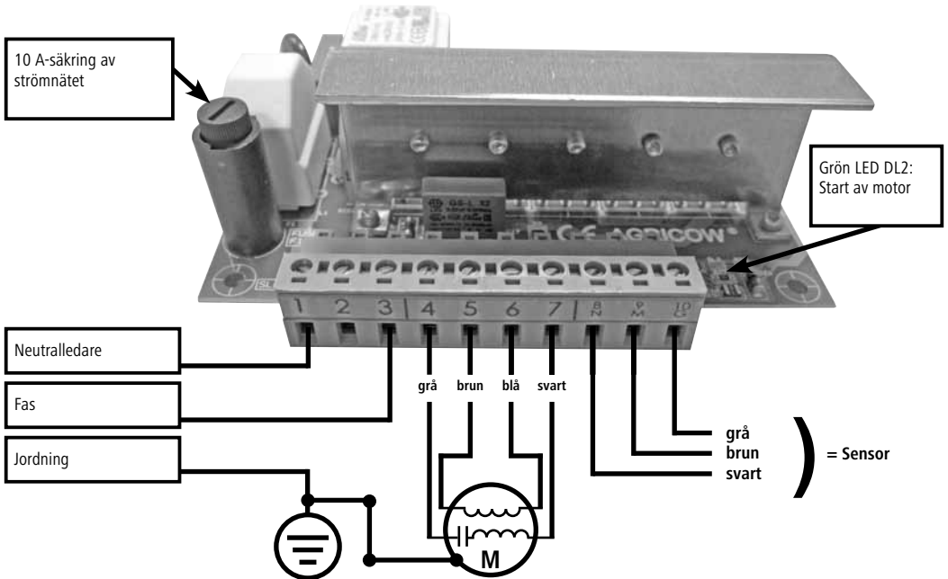
Bild 5.2: Anslutningsbild för CowCleaner Swing t.o.m. 2015
