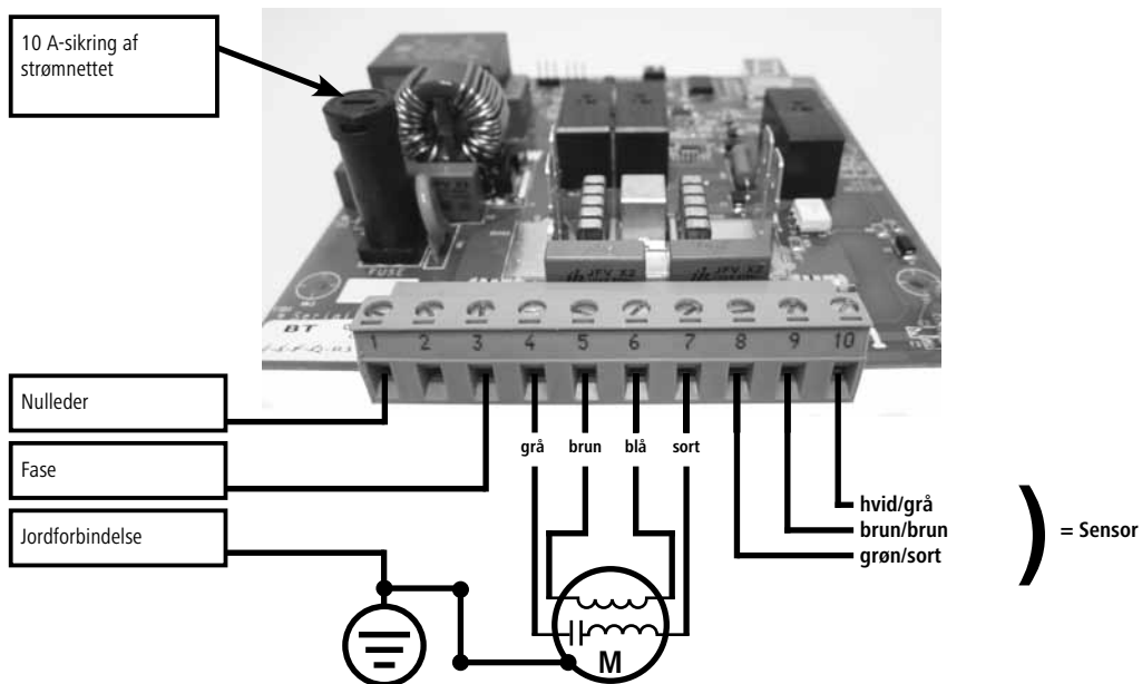
Illustration 4.2: Tilslutningsbillede for CowCleaner Swing indtil 2015
