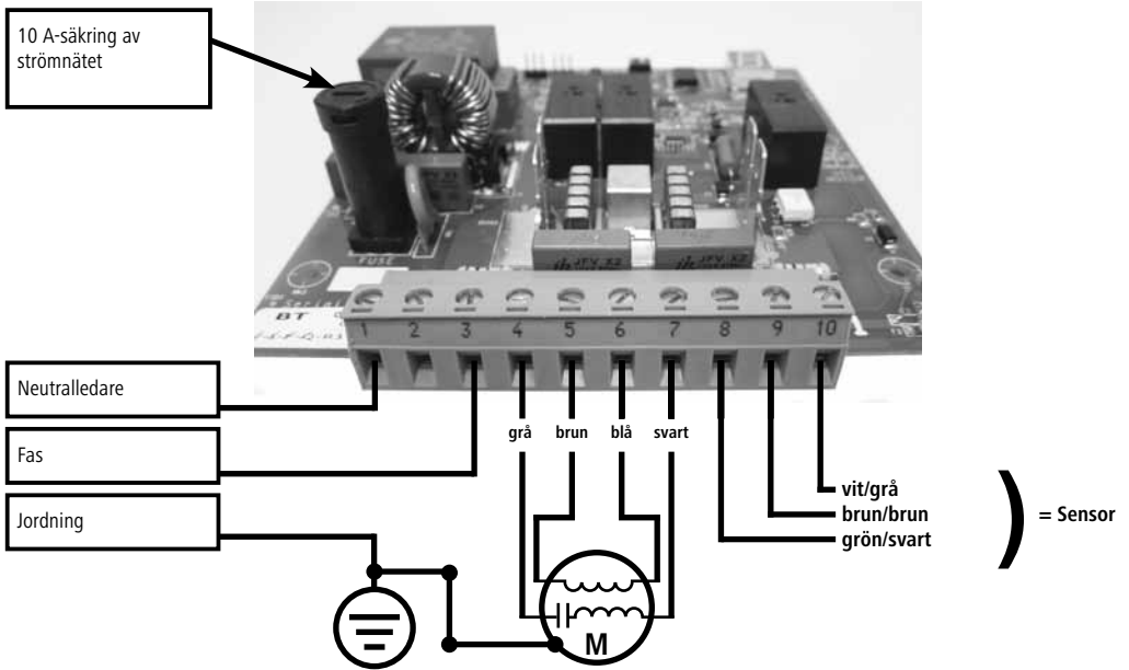
Bild 5.2: Anslutningsbild för CowCleaner Swing t.o.m. 2015
