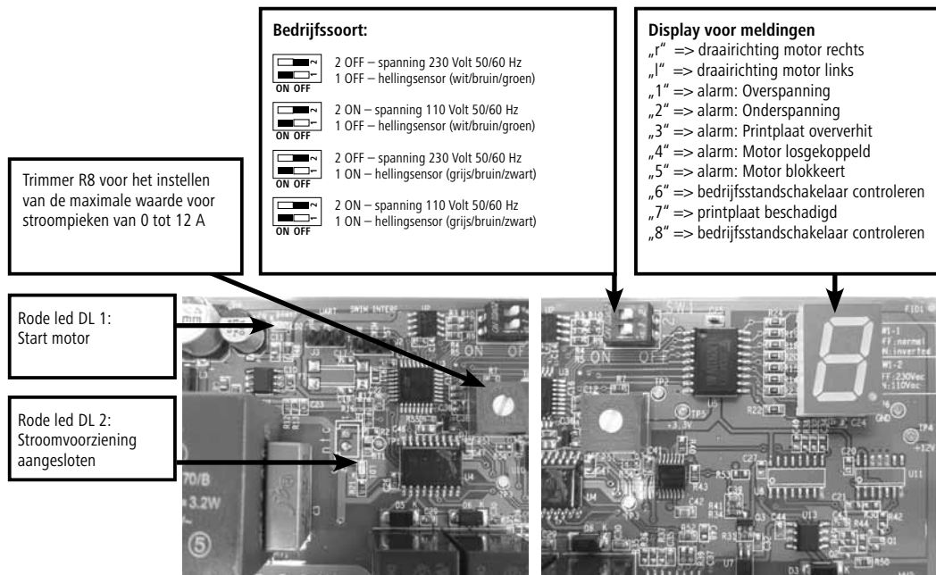
Afbeelding 4.2: Printplaat voor CowCleaner Swing vanaf 2015
