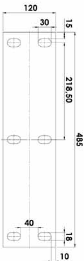
Abbildung 2: Lochbild
