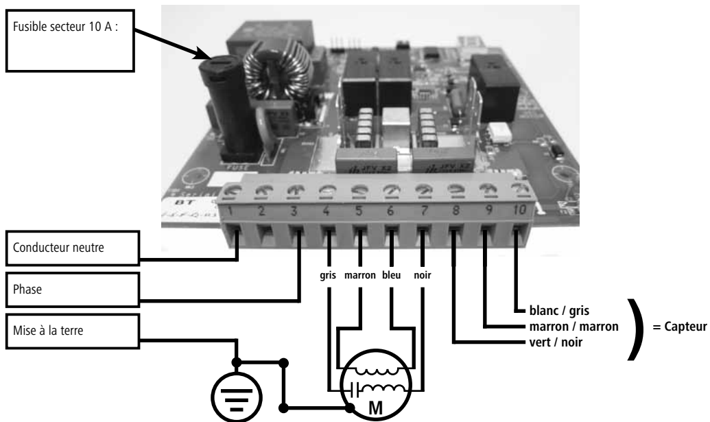
Figure 5.2 : schéma de raccordement pour CowCleaner Swing jusqu'en 2015
