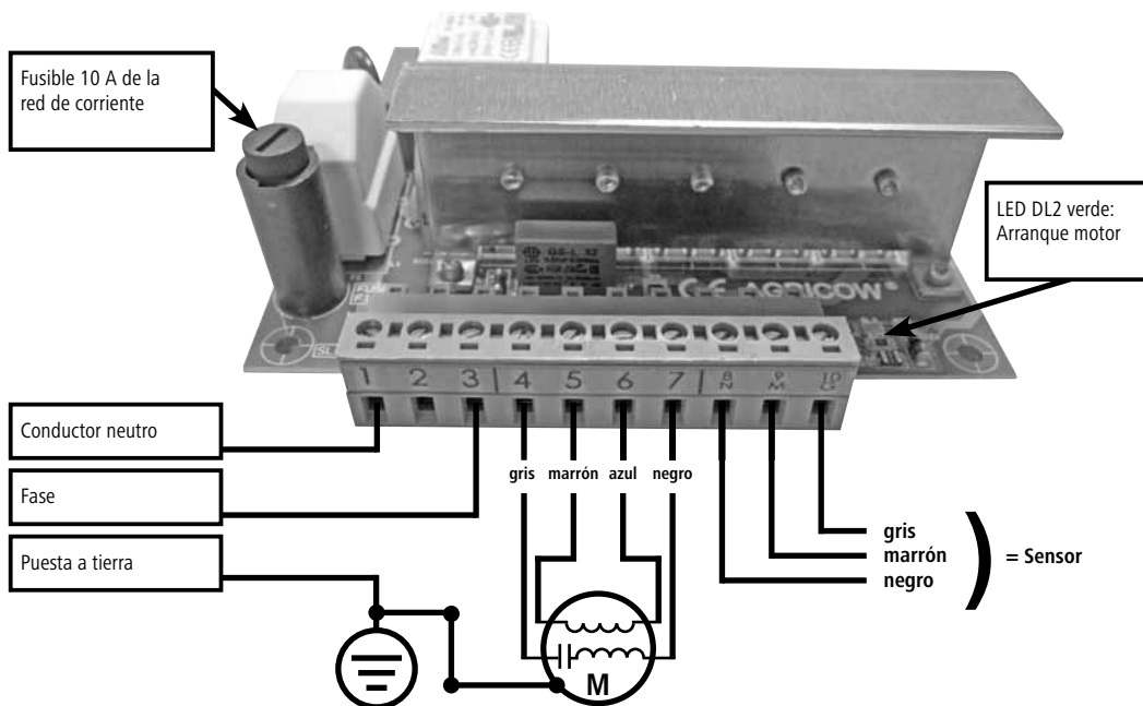
Figura 5.2: Esquema de conexiones para CowCleaner Swing hasta 2015
