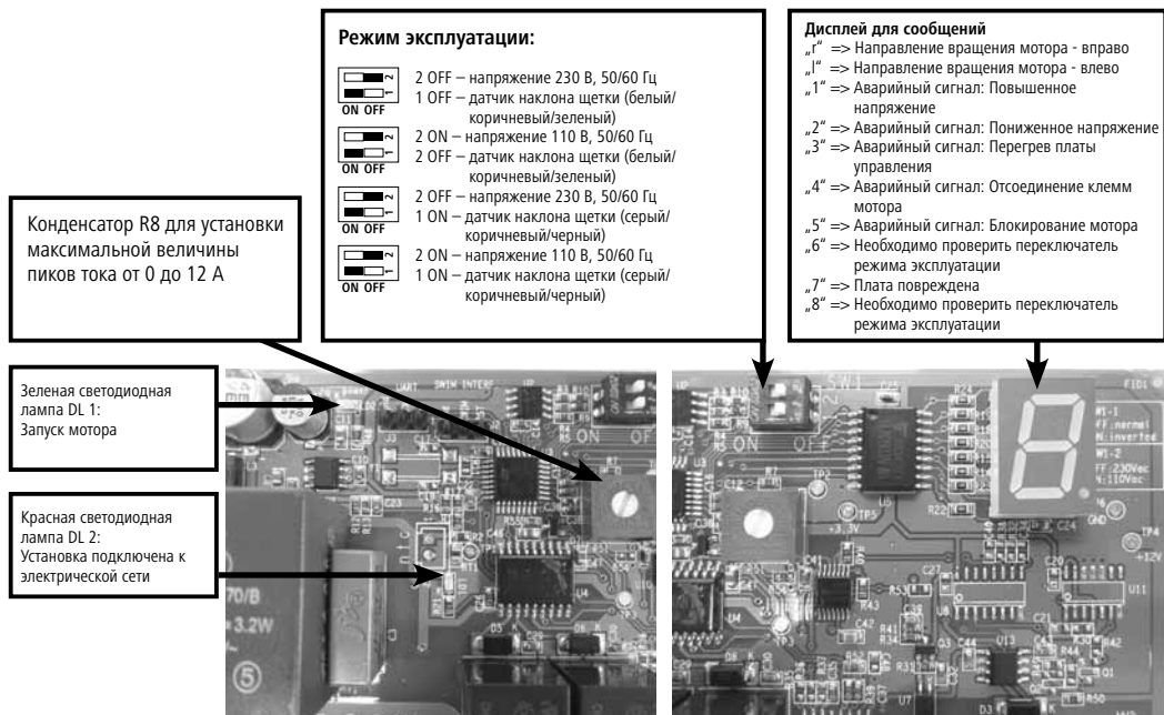
Рисунок 4.2: Плата CowCleaner Swing до 2015 г.
