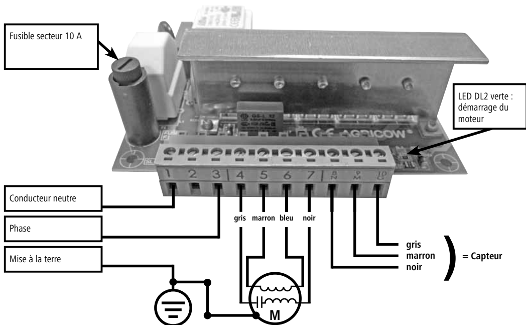
Figure 5.2 : schéma de raccordement pour CowCleaner Swing jusqu'en 2015
