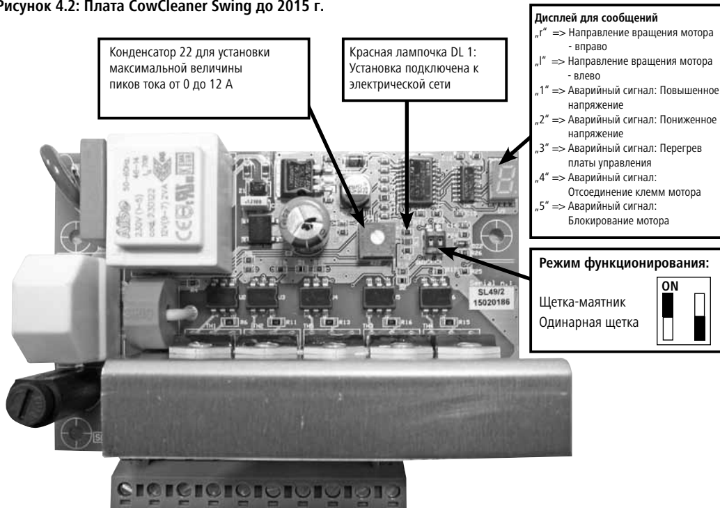
Рисунок 4.2: Плата CowCleaner Swing до 2015 г.
