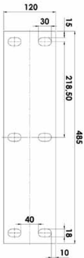
Bild 2: Hålbild
