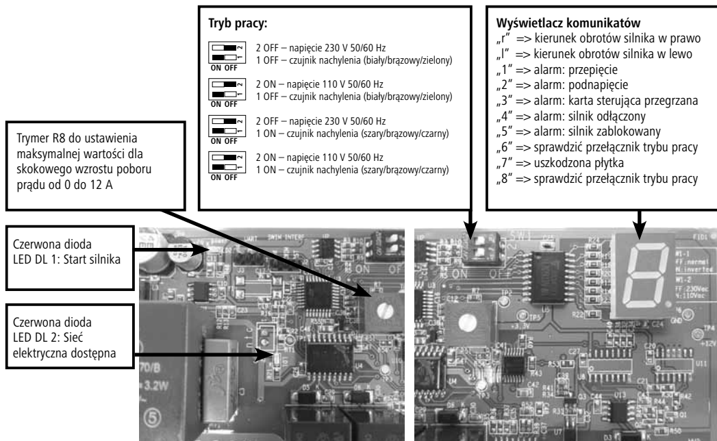
Rysunek 4.2: Płytki obwodu drukowanego do CowCleaner Swing od 2015
