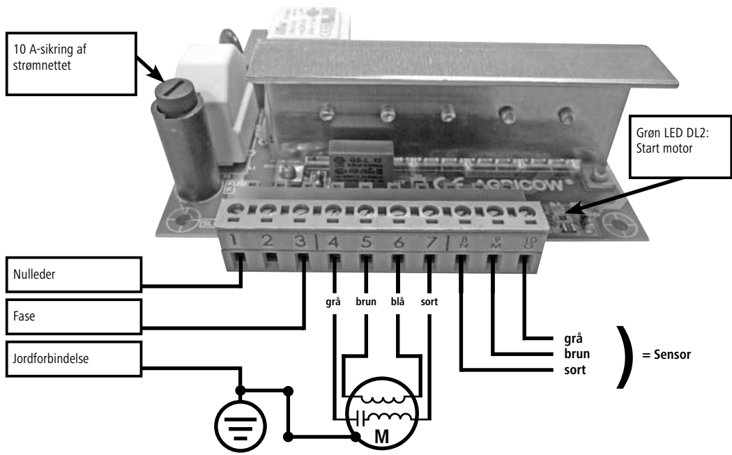
Illustration 4.2: Tilslutningsbillede for CowCleaner Swing indtil 2015
