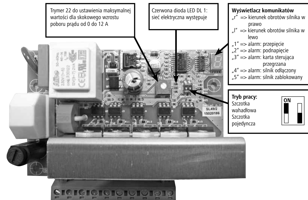
Rysunek 4.2: Płytki obwodu drukowanego do CowCleaner Swing od 2015
