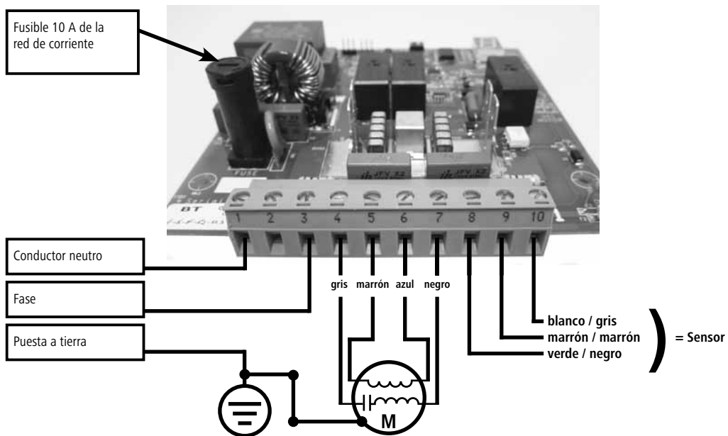
Figura 5.2: Esquema de conexiones para CowCleaner Swing hasta 2015
