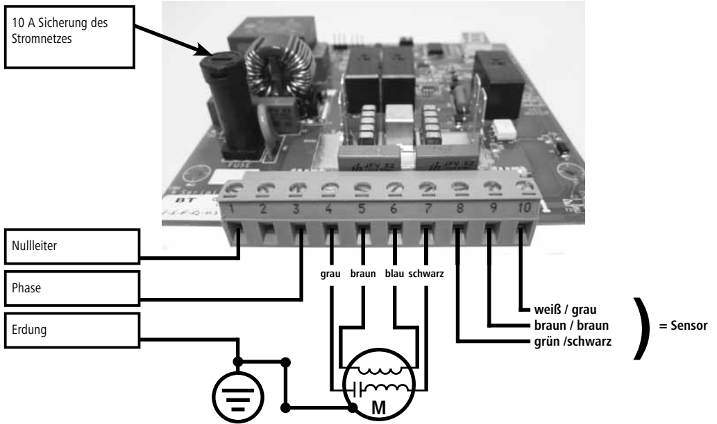
Abbildung 5.2: Anschlussbild für CowCleaner Swing bis 2015
