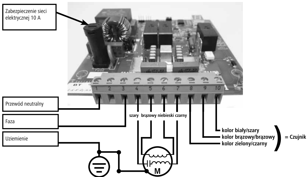
Abbildung 5.2: Anschlussbild für CowCleaner Swing bis 2015
