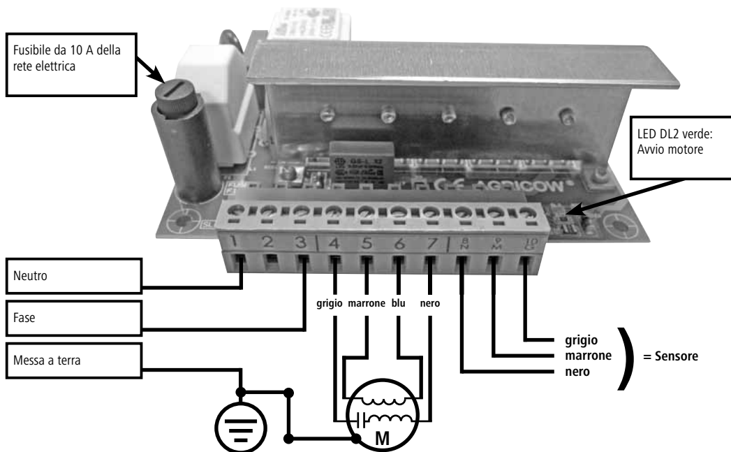
Figura 5.2: Schema dei collegamenti per CowCleaner Swing fino al 2015
