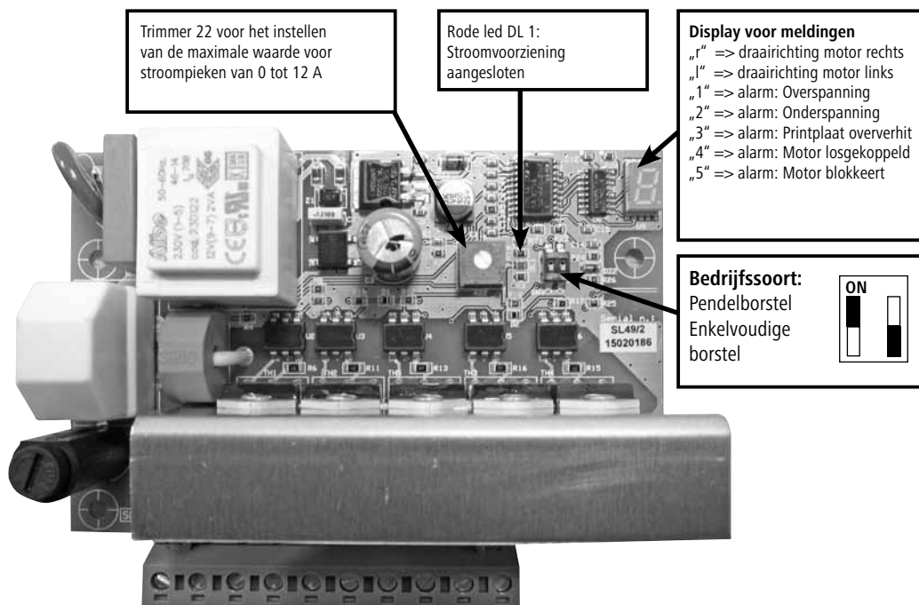
Afbeelding 4.2: Printplaat voor CowCleaner Swing vanaf 2015
