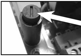
Abbildung 6: Sicherungswechsel für CowCleaner Swing
