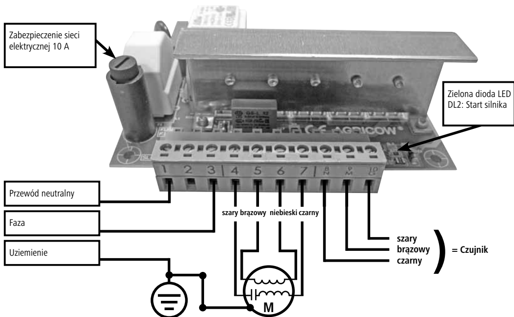
Abbildung 5.2: Anschlussbild für CowCleaner Swing bis 2015
