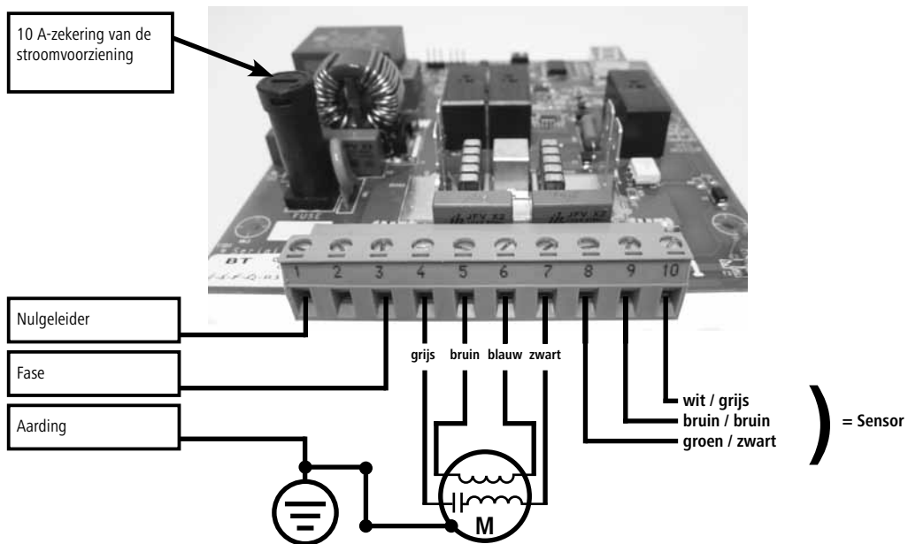
Afbeelding 5.2: Aansluitschema voor CowCleaner Swing tot 2015
